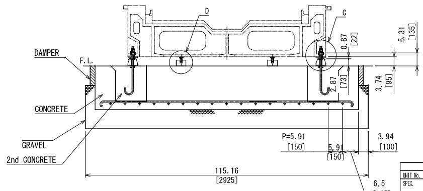
A-A SECTION
