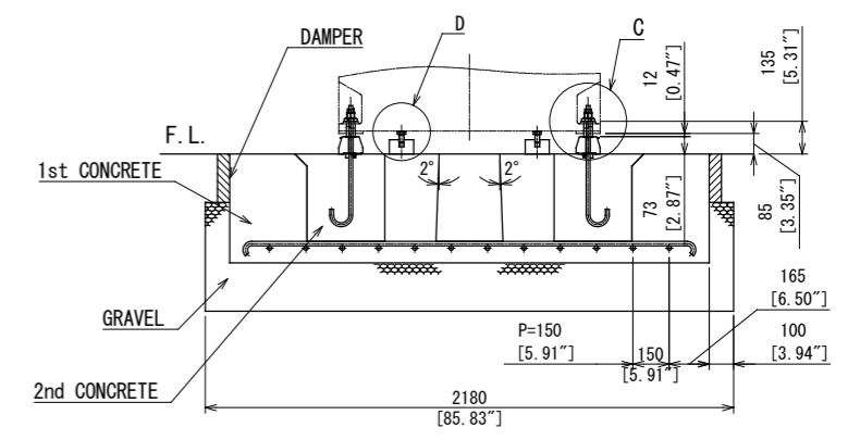
A-A SECTION
